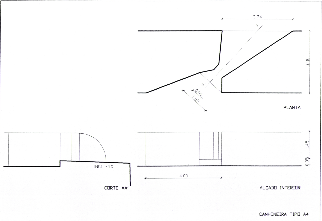
FIG.46- FORTALEZA DE MAZAGÃO / LEVANTAMENTO DAS CANHONEIRAS SUPERIORES CANHONEIRA TIPO A3 / CANHONEIRAS 13, 15, 17, 56, 59, 60 FIG.47- FORTALEZA DE MAZAGÃO / LEVANTAMENTO DAS CANHONEIRAS SUPERIORES CANHONEIRA TIPO A4 / CANHONEIRA 64.
