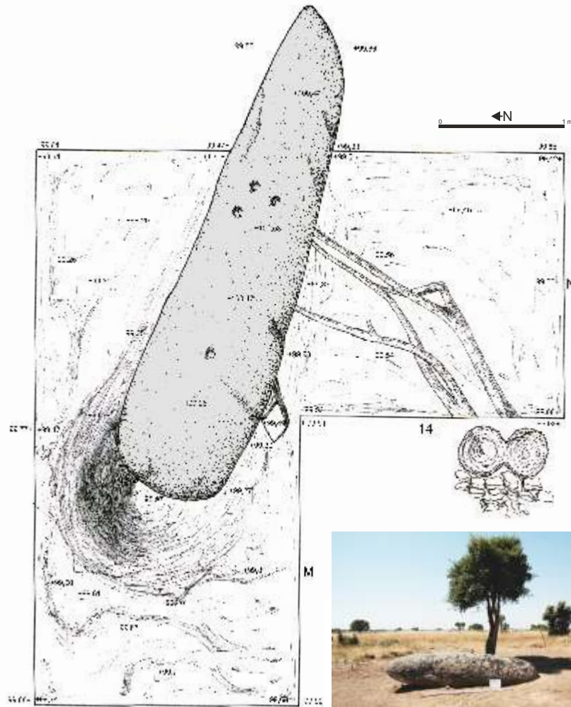
Menhir do Patalou, área escavada
