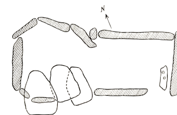
Anta 2 dos Saragonheiros. (Desenho: George e Vera Leisner, 1959)
