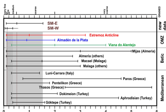
Figura 9. Comparación de la granulometría entre las muestras de mármol estudiadas y otros mármoles de Hispania y del Mediterráneo explotados en época romana (granulometría adaptada de Lapuente, 1995; Lapuente y Turi, 1995; Antonelli y Lazzarini, 2015).
