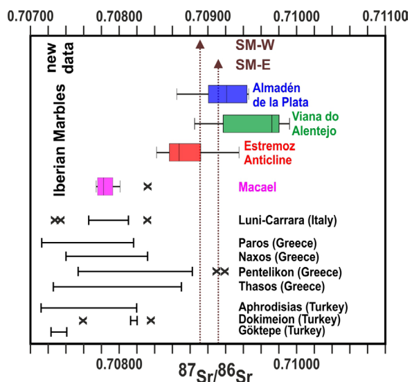
Figura 8. Firma isotópica de estroncio de los mármoles blancos utilizados en los capiteles de la Iglesia de Santa María Magdalena y comparación con los valores obtenidos en mármoles ibéricos y otros mármoles mediterráneos significativos (valores bibliográficos ^{87}\text{Sr}/^{86}\text{Sr} adaptados de Brilli, Cavazzini y Turi, 2005; Morbidelli et al. , 2007; Zöldföldi, 2011; Taelman et al. , 2013; Moreira et al. , 2019, 2020; Wielgosz-Rondolino et al. , 2020). Nótese que la relación isotópica obtenida por ambas muestras es compatible con los mármoles de la OMZ (Anticinal de Estremoz, Viana do Alentejo y Almadén de la Plata) y Pentélico (Grecia).
