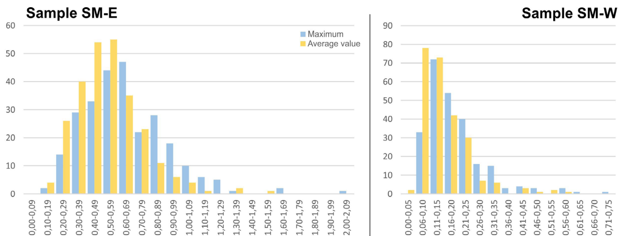
Figura 4. Distribución del tamaño del grano de calcita en las muestras estudiadas (elaborado por N. Moreira).
