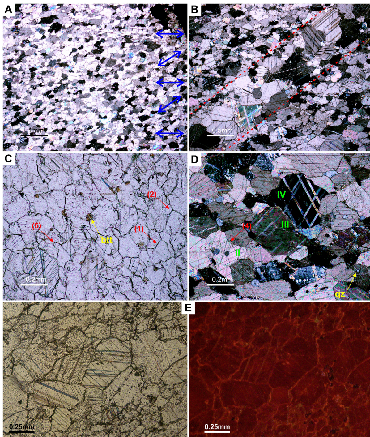
Figura 6. Características petrográficas de la muestra SM W (Capitel 2): (A) vista general de la textura homeoblástica orientada (nícoles cruzados); (B) vena de grano medio de calcita cortando el mármol de grano fino (nícoles cruzados); (C) y (D) mineralogía, maclas de calcita y forma de los límites de calcita - (1) rectos, (2) poligonales, (3) suturados, (4) curvados, (5) embebidos (c - nicols paralelos y d - nicols cruzados); (E) facies de catodoluminescencia mostrando distinto comportamiento entre los bordes y el interior de los granos de calcita (tiempo de exposición de 3 segundos) (elaborado por N. Moreira).
