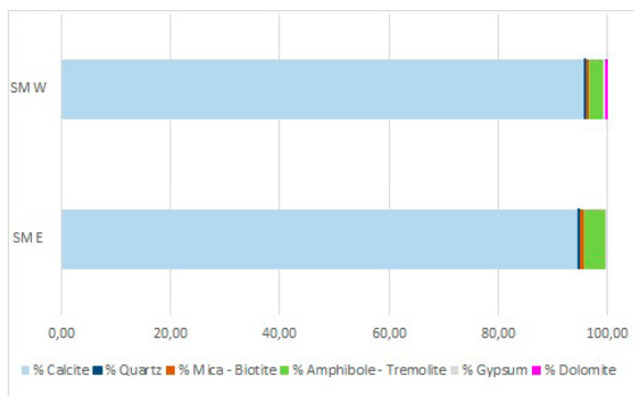
Figura 7. Composición mineralógica de los mármoles blancos utilizados en los capiteles de la iglesia de Santa María Magdalena mediante el análisis DRX (elaborado por N. Moreira).
