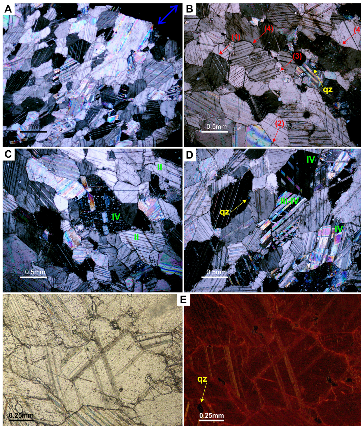
Figura 5. Características petrográficas de la muestra SM E (Capitel 1): (A) vista general de la textura heteroblástica orientada; (B) forma del límite de la calcita - (1) recto, (2) poligonal, (3) suturado, (4) curvado, (5) incrustado; (C) y (D) (todas las microfotografías presentadas se obtuvieron con nicols cruzados); (E) facies de catodoluminiscencia mostrando distinto comportamiento entre los bordes y el interior de los granos de calcita (tiempo de exposición de 3 segundos) (elaborado por N. Moreira).
